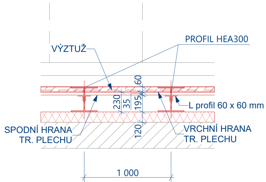
DETAIL - HORNÍ HRANA TR. PLECHU
