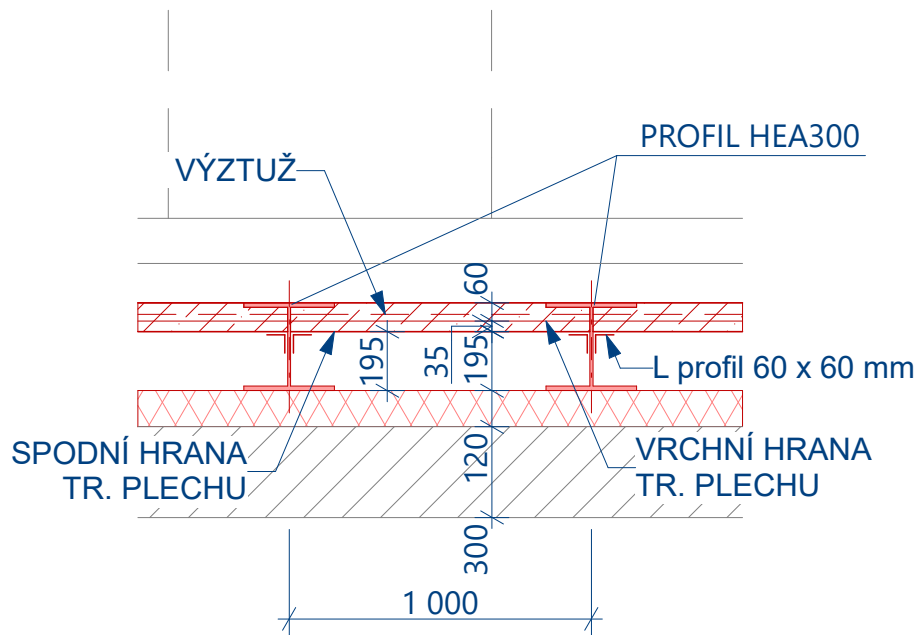
DETAIL - SPODNÍ HRANA TR. PLECHU
